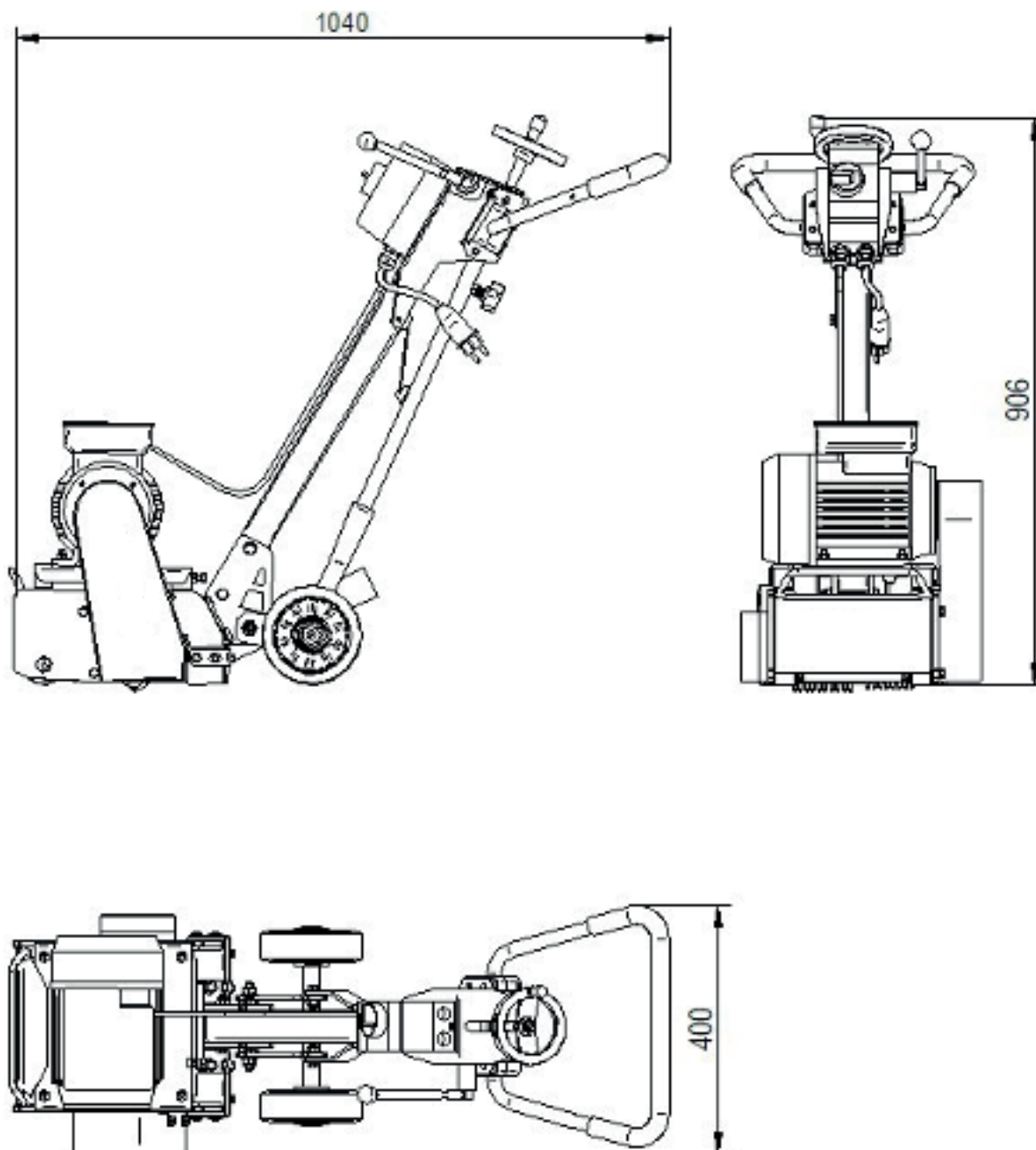
Dimensioni della fresatrice SCARIMAX 200
