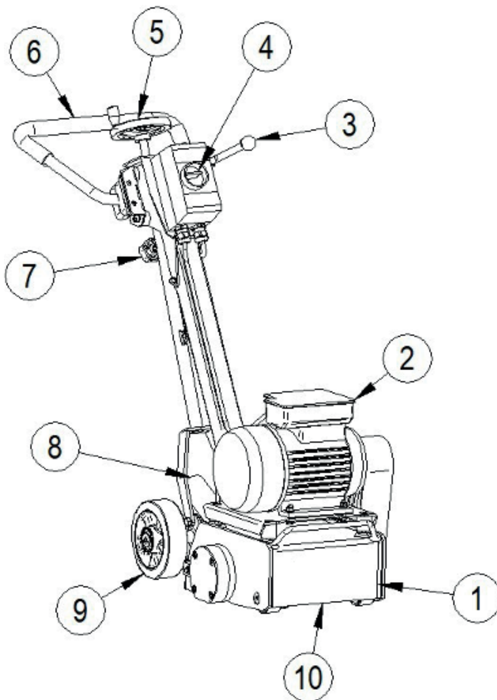
Parti funzionali della fresatrice SCARIMAX 200
