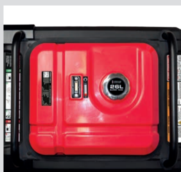
Serbatoio e indicatore livello carburante
