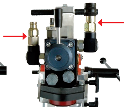
Ingresso ed uscita olio idraulico
