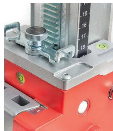
Doppia livella e leva per arresto calata
