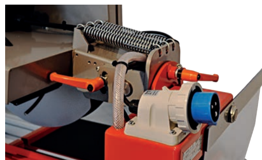
Monofase, tripla molla per un'agile basculanza
