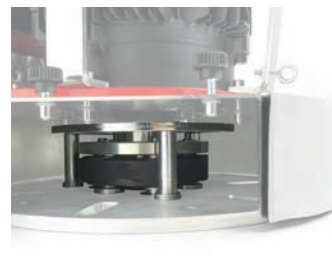
Cuscinetto in gomma per una migliore aderenza al pavimento ed una riduzione delle vibrazioni
