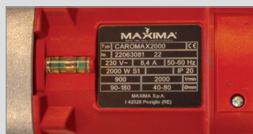
Bolla inclinazione ed informazioni complete
